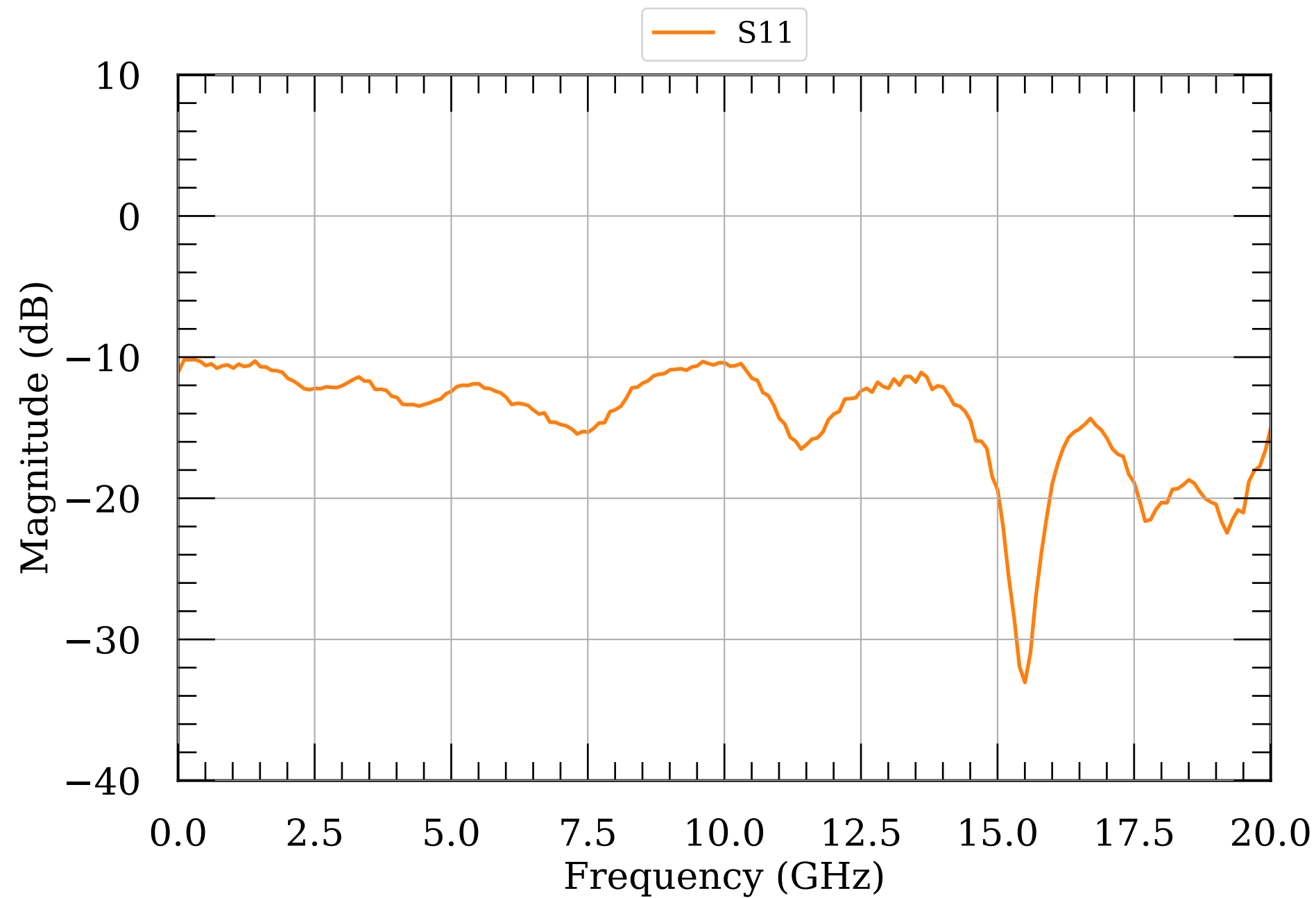
LNA S-params module007
